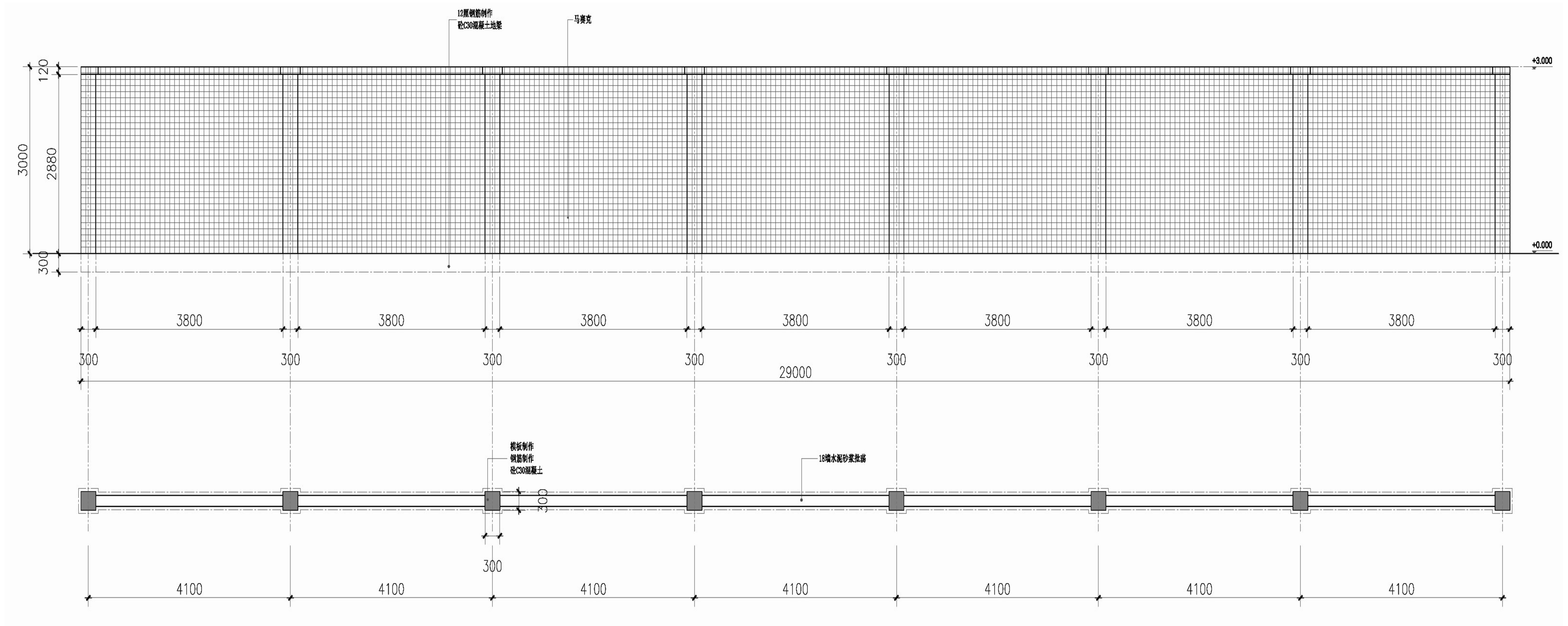
清远市妇幼保健院北院墙重砌段大样图
